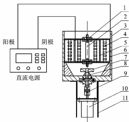
1—支架;2—圆柱棒状阳极;3—槽体;4—泡沫镍三维粒子电极;5—泡沫镍阴极板;6—圆筒状阳极;7—叶轮;8—密封圈;9—联轴器;10—电机;11—电机支座。
