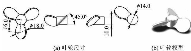
图6 叶轮模型
