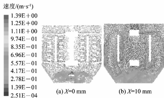
图11 X=0 mm 和 X=10 mm 截面速度矢量图
