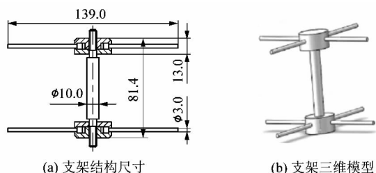
图4 支架模型
