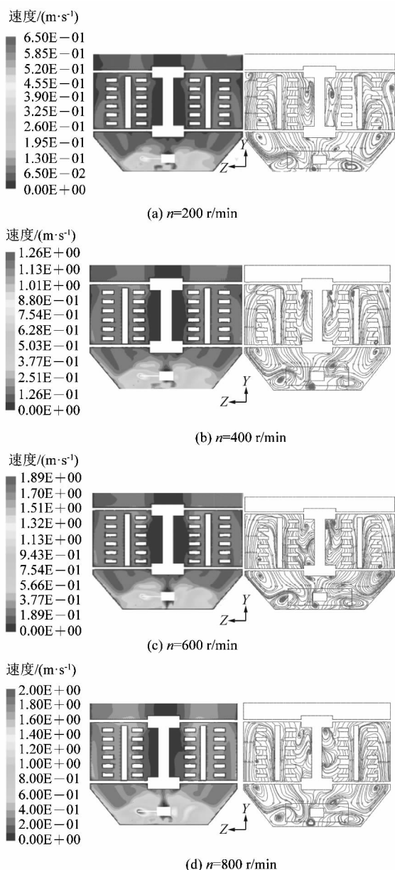
图9 不同转速时 X=0 mm 截面速度云图和迹线图
