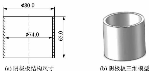
图5 阴极板模型
