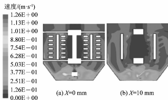
图10 X=0 mm 和 X=10 mm 截面速度云图
