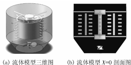
图8 流体模型
